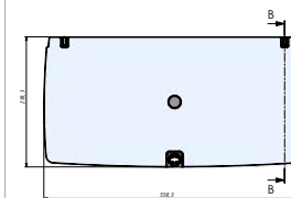
Kookplaat TAI55MD Afmetingen: 558,3x278,3 mm
